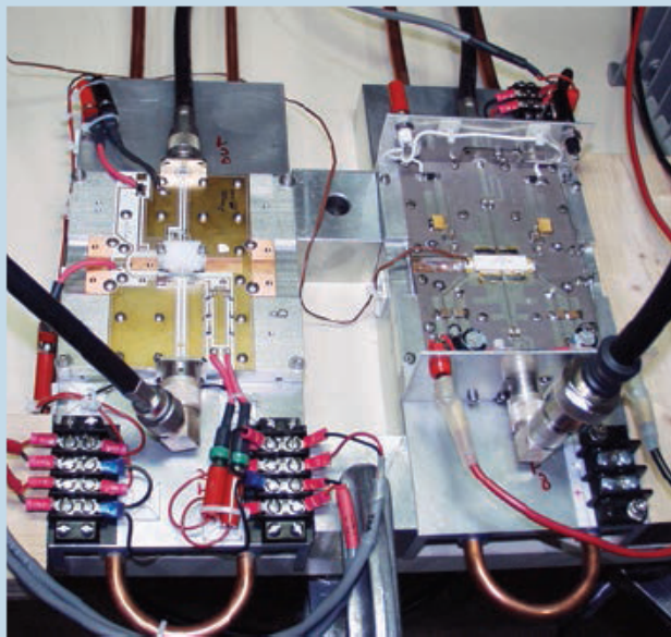
S-band 150-W CW rf amplifier
